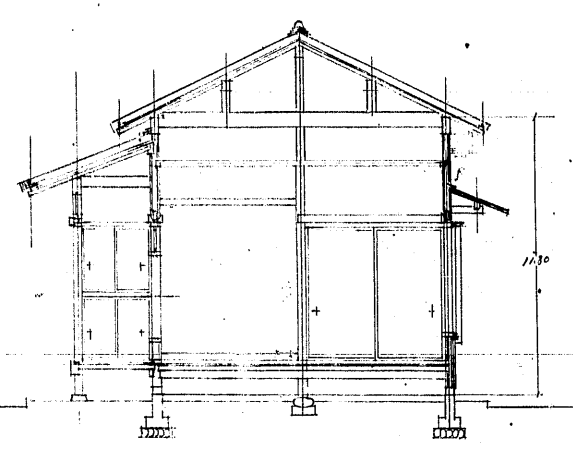
八形縦断面図
