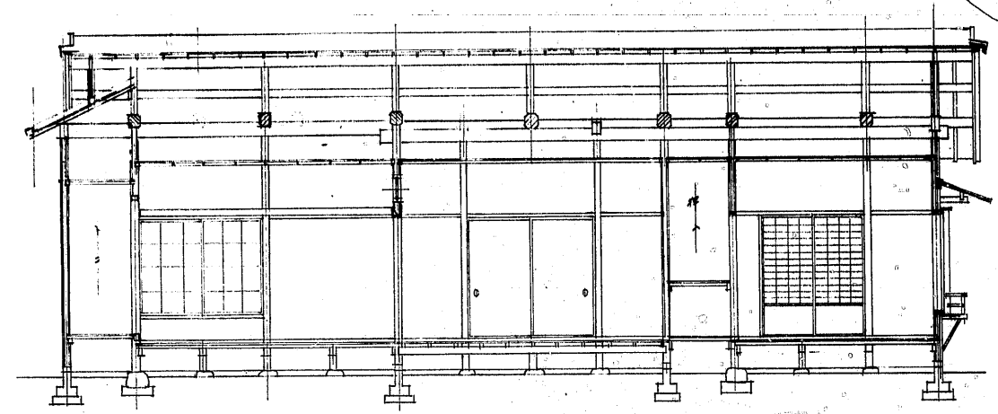
横断面図
