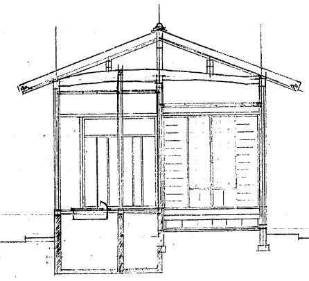
三間棟断面図
