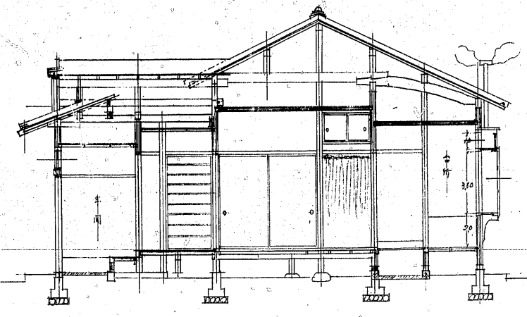
五間四柱米台所縦断面図
