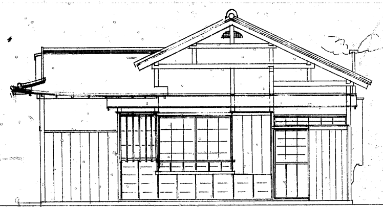
東側等図
