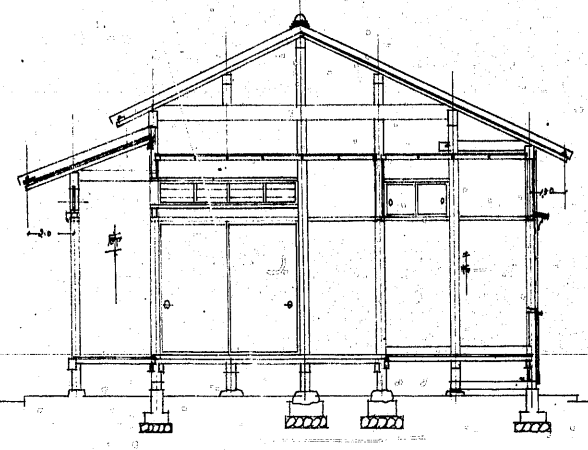
六形六柱縦断面図
