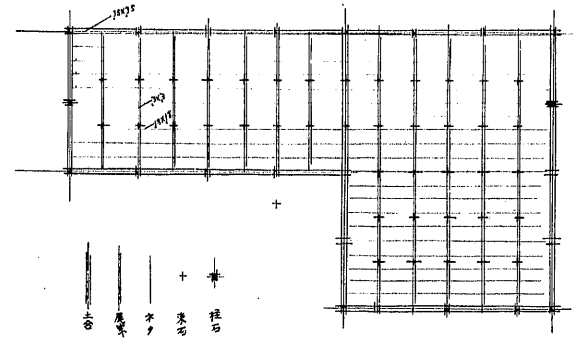
地敷及床伏圖
