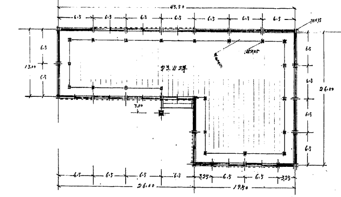
平面圖 1/100
