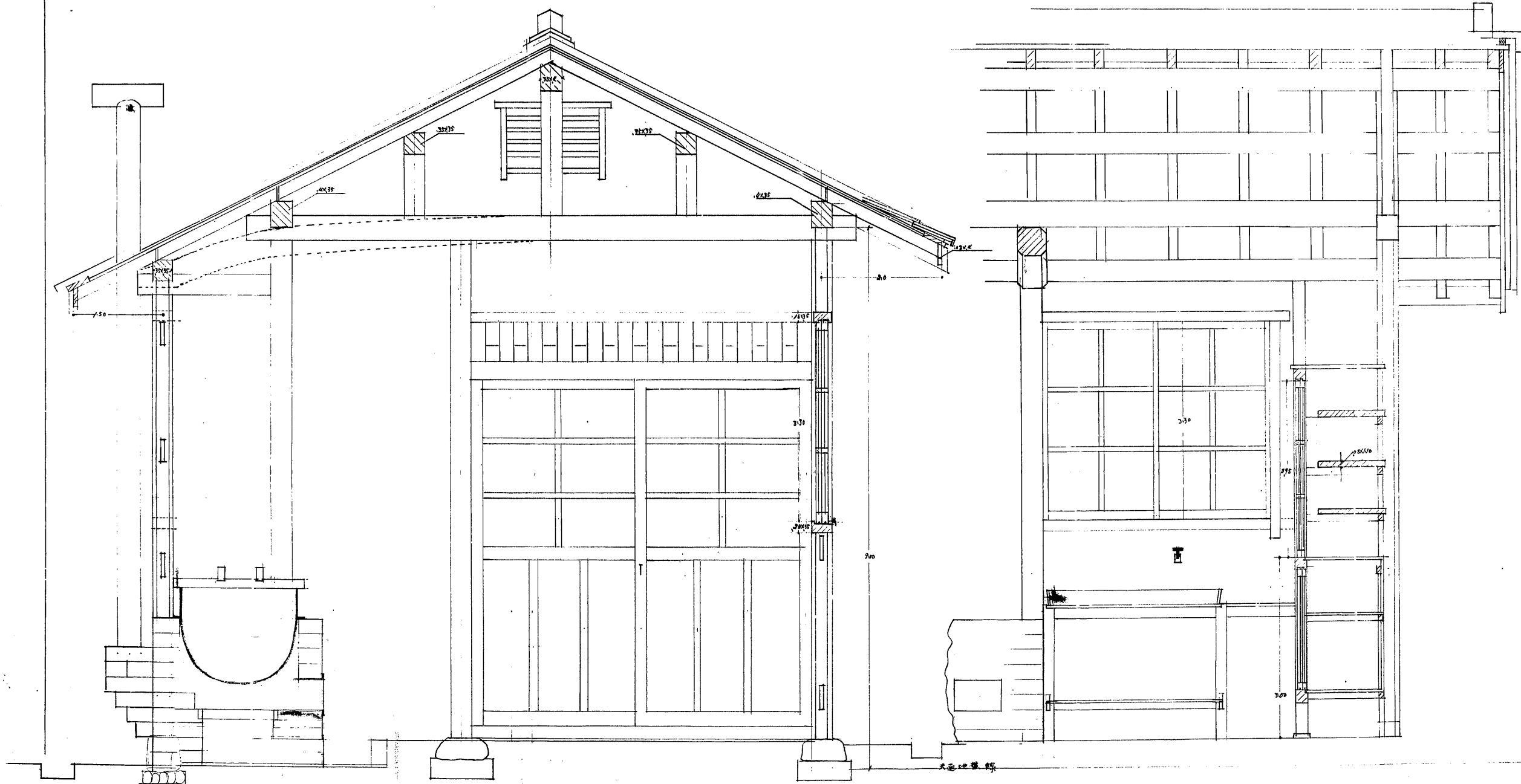
湯沸場縦断
