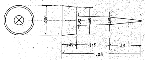
16 脇門扉入双金物止釘
