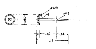
13 脇門扉板止釘
