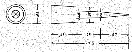
17 大扉入刃金物止鉄
