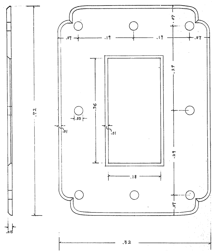
② 肘重座金
