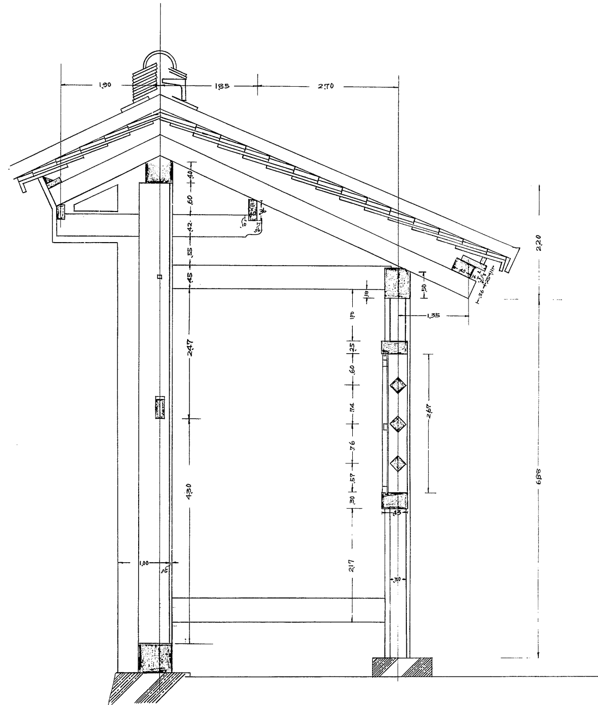
旧番所 断面
