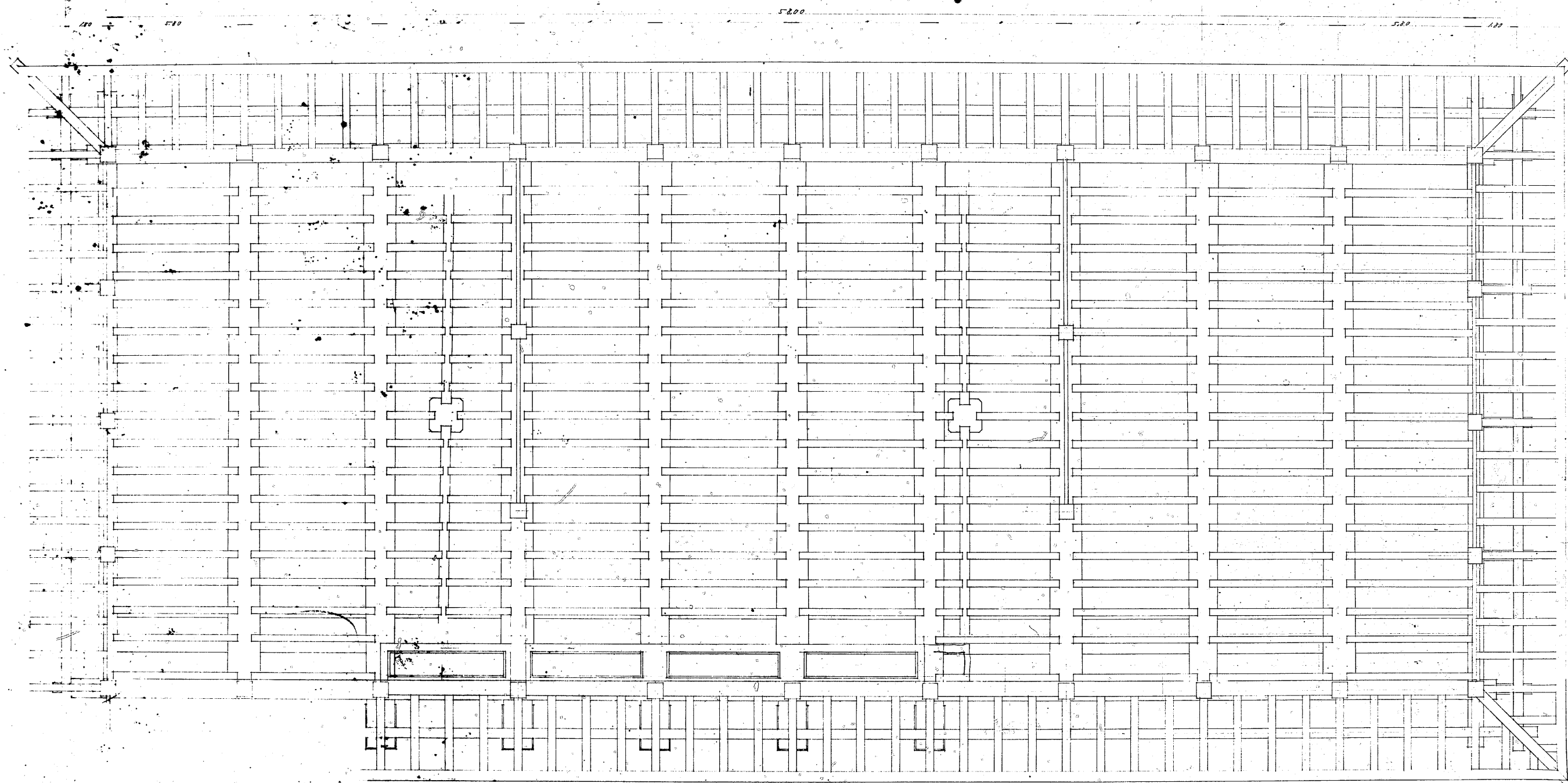
第二階床伏図 縮尺 1/20
