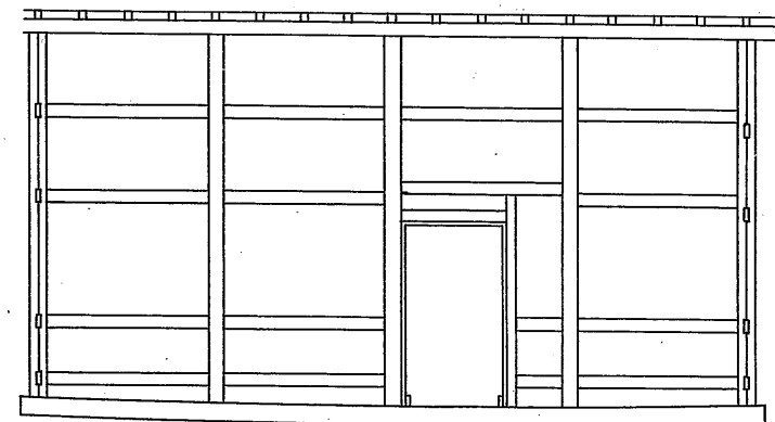
イ立面
