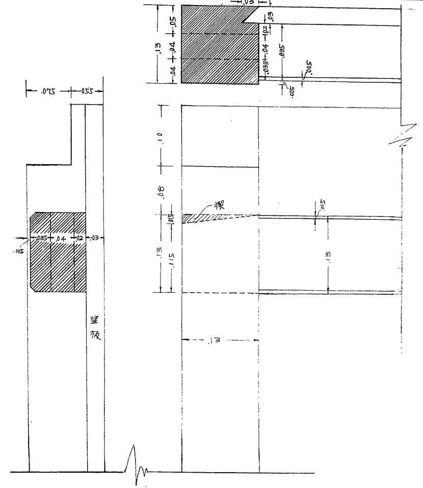
板戸仕口詳細(廻)
