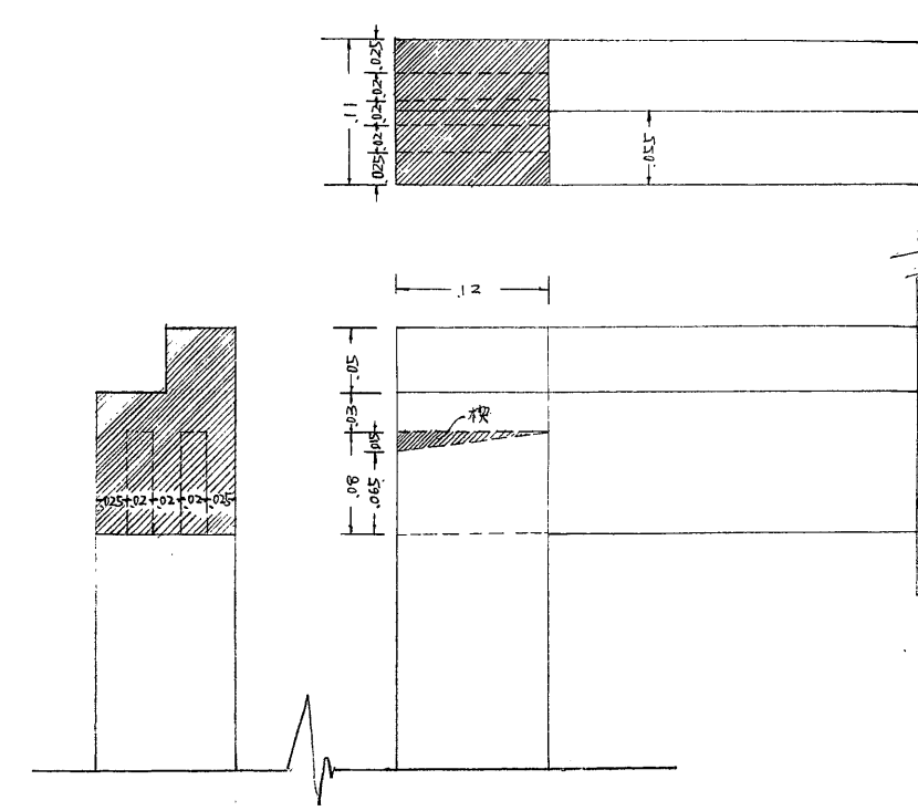
障子仕口詳細(廻)
