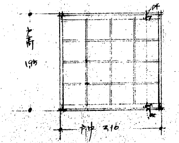
下地窓部矩計
