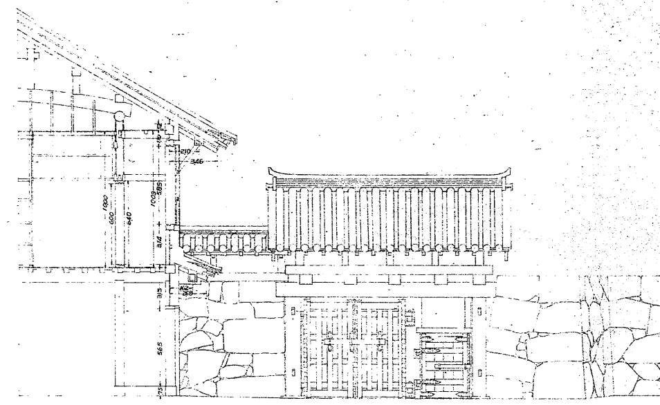
G-G 立面
