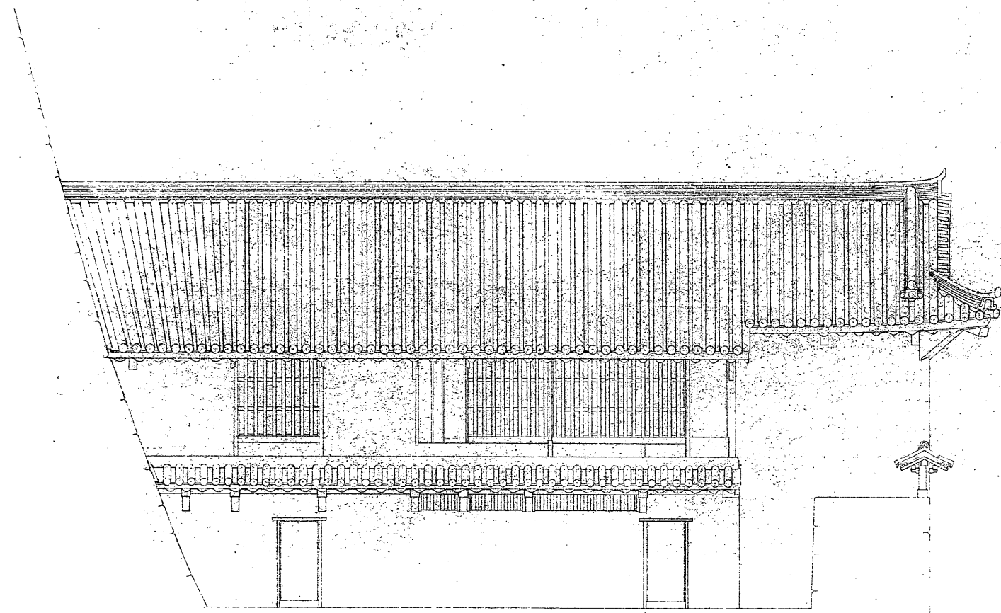
F-F 立面
