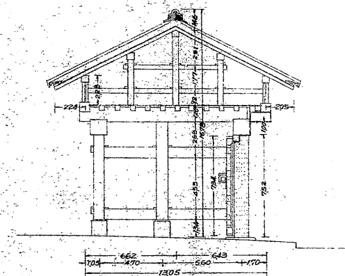
B—B 断面
