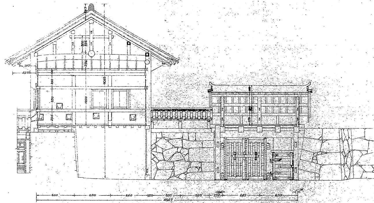
A—A 断面
