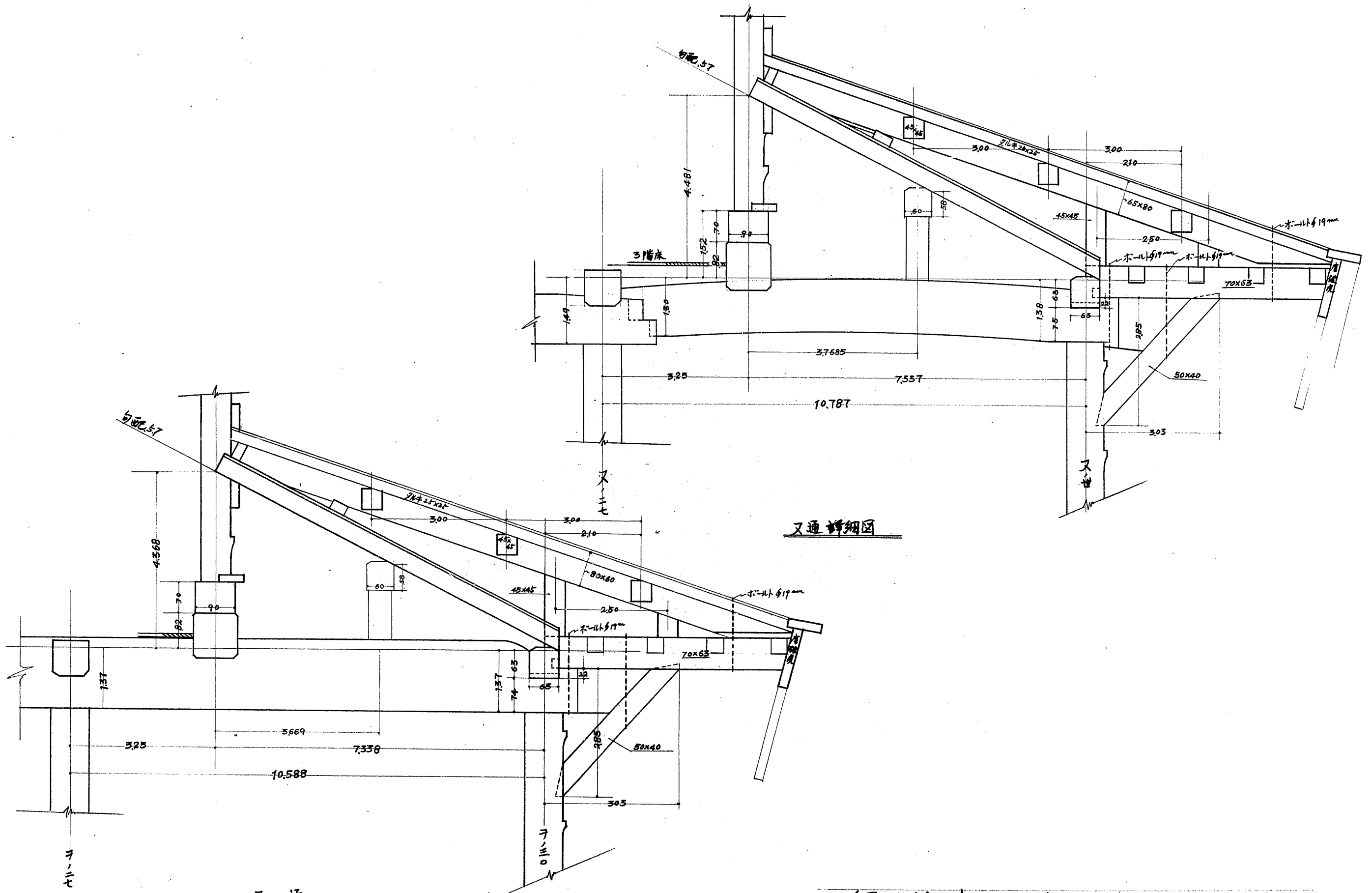
姫路城乾小沃寺3階床梁施工図 5/20
