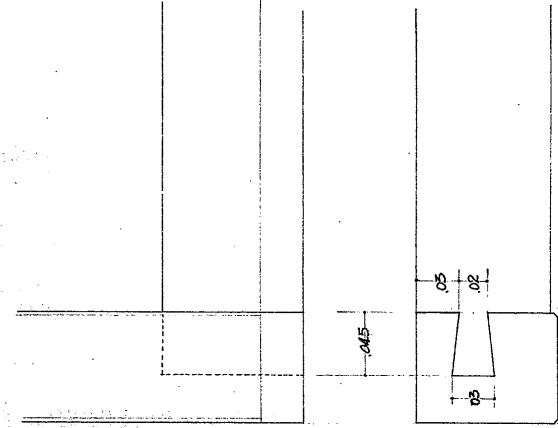
框組手現寸図
