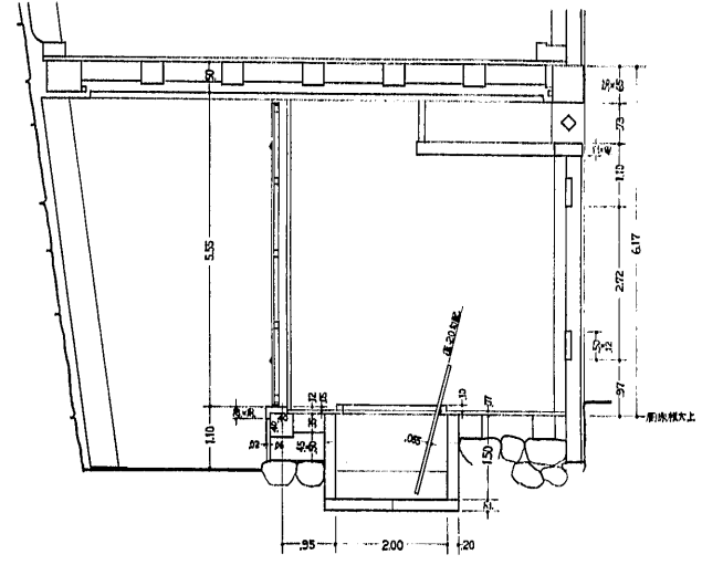
横断面
