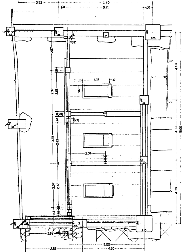
平面
