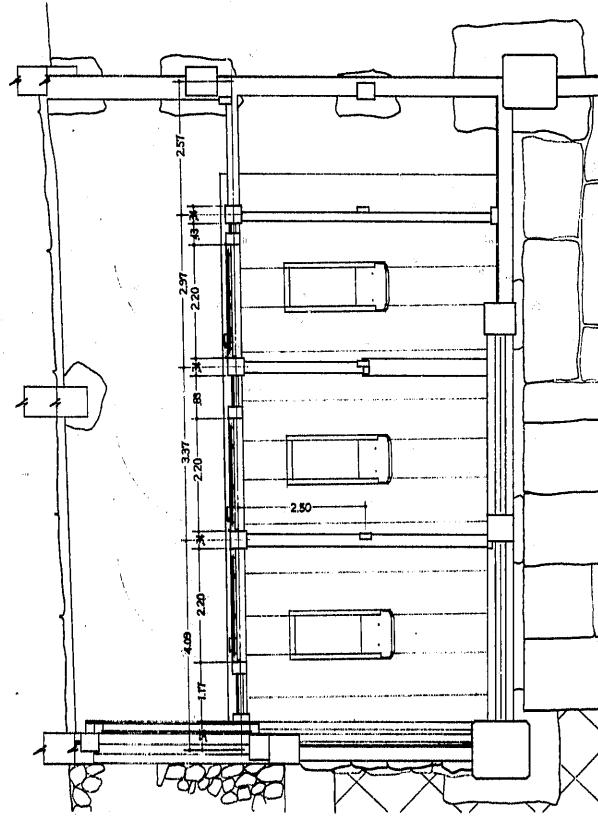
修理前平面
