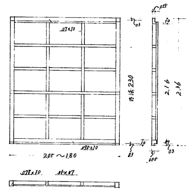
2階側窓板戸 1*
