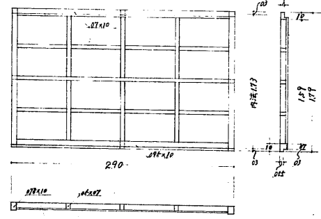
2階側窓板戸 2*
