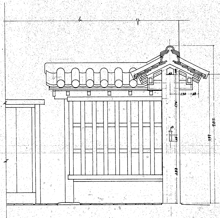
土堀前面と武家立面図
