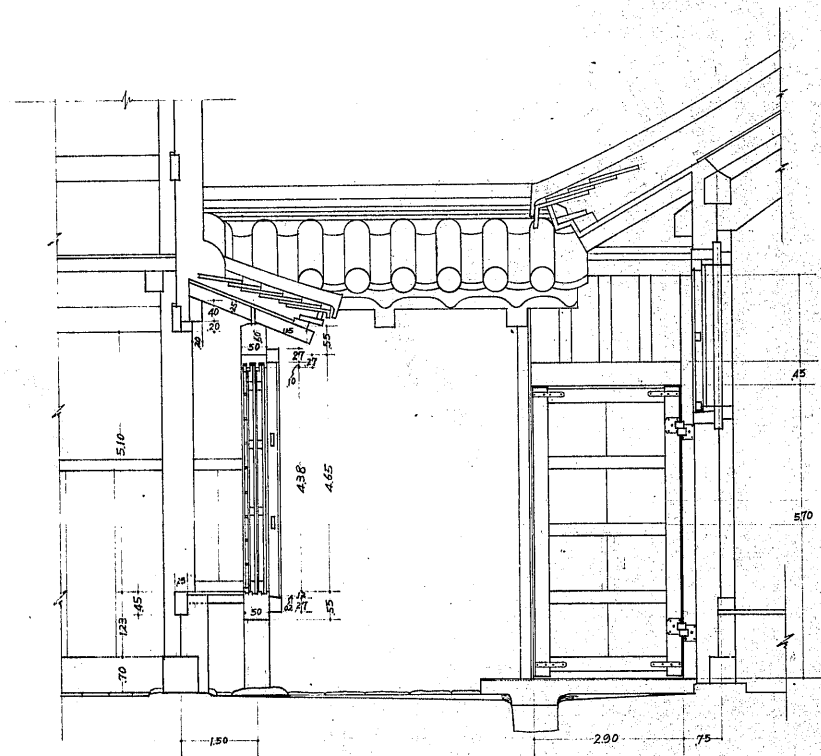
武家断面と土堀北側立面図
