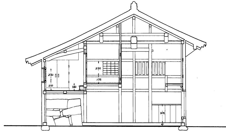
A~A' 断面
