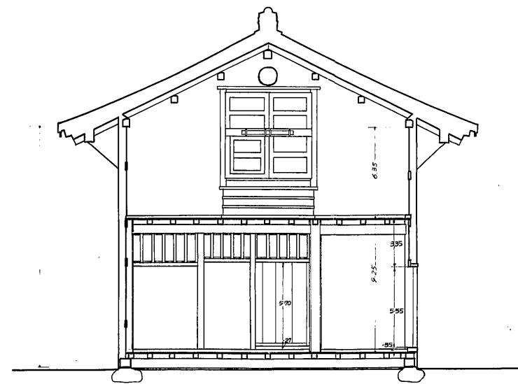
D~D' 断面
