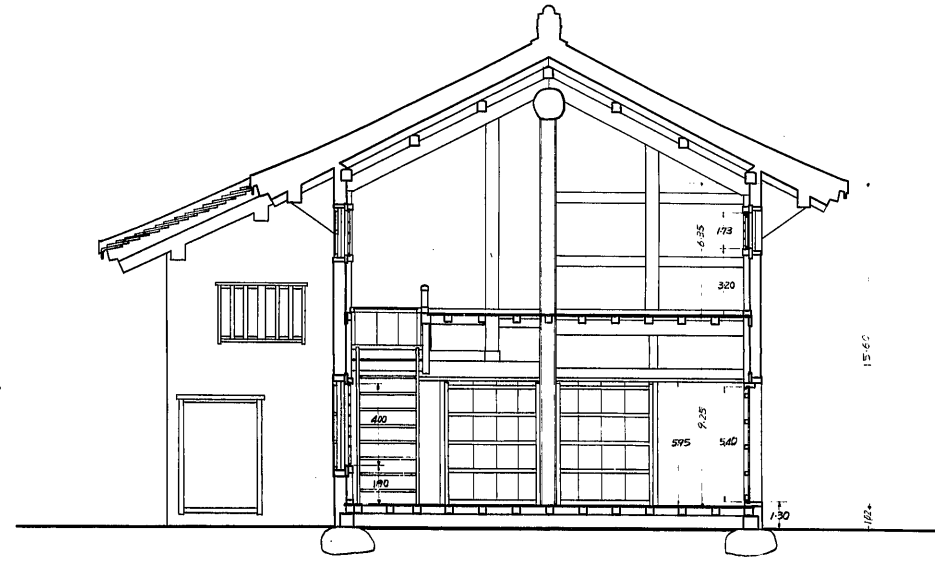
C~C' 断面
