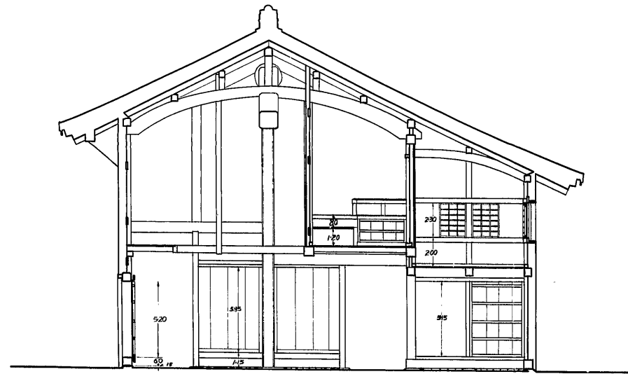
B~B' 断面
