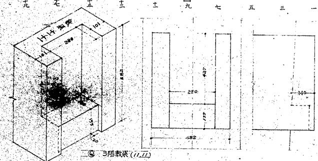
(D) 3階梁開口図 (1/100)
