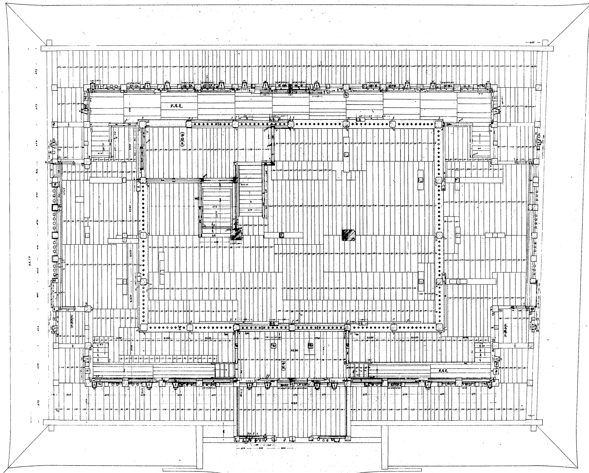
参階平面図 1/50
