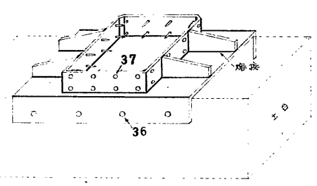
柱根巻上台敷金具 (29)
