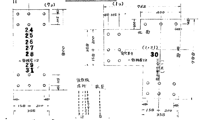
上台敷金具南強敷鉄板
