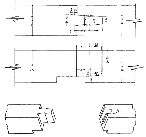
3. 床梁継手
