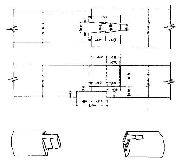
2. 床梁継手
