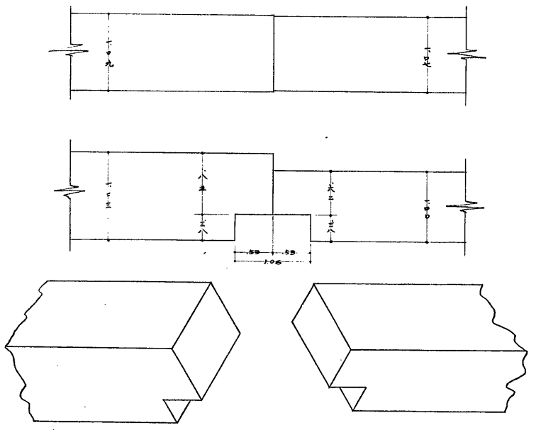
4. 床梁継手
