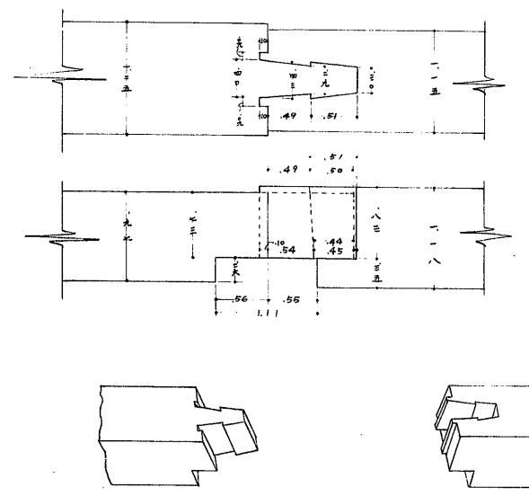
1. 床梁継手
