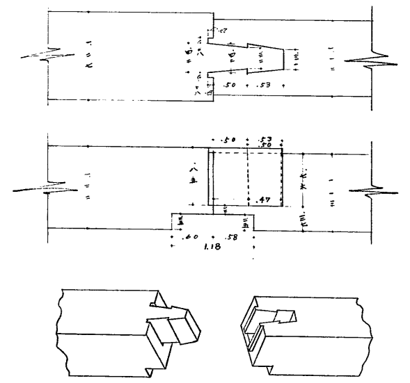
5. 床梁継手
