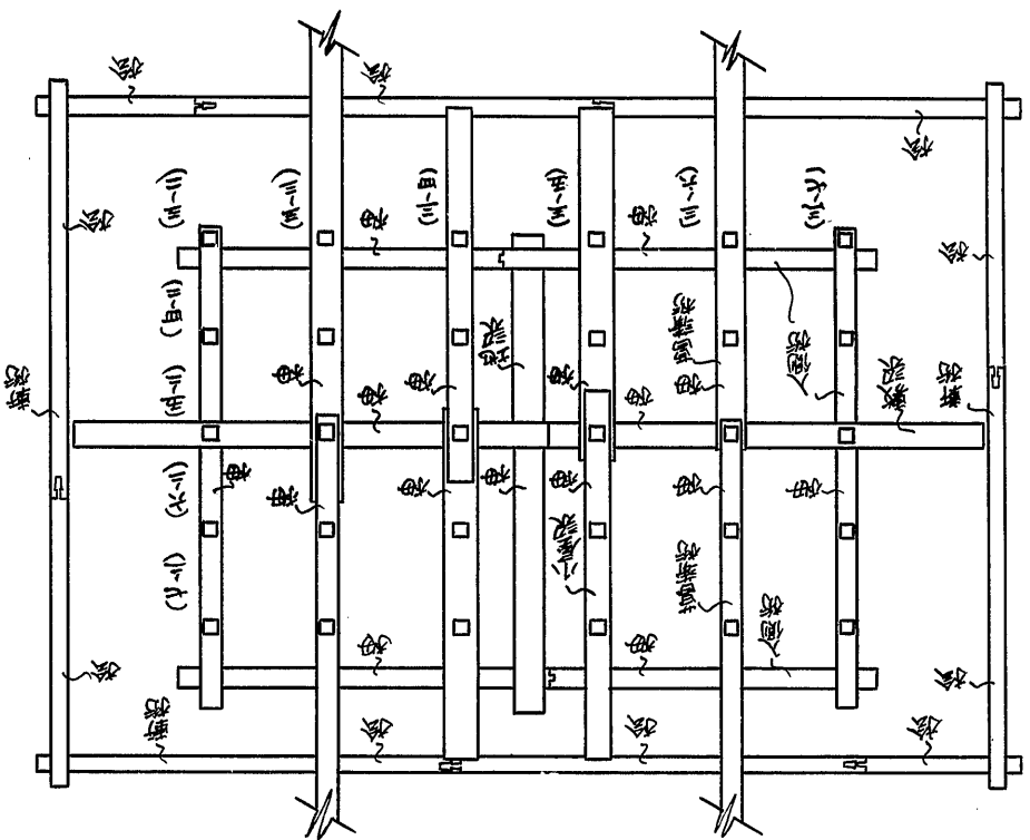
特級忍風堂の梁架配置図
